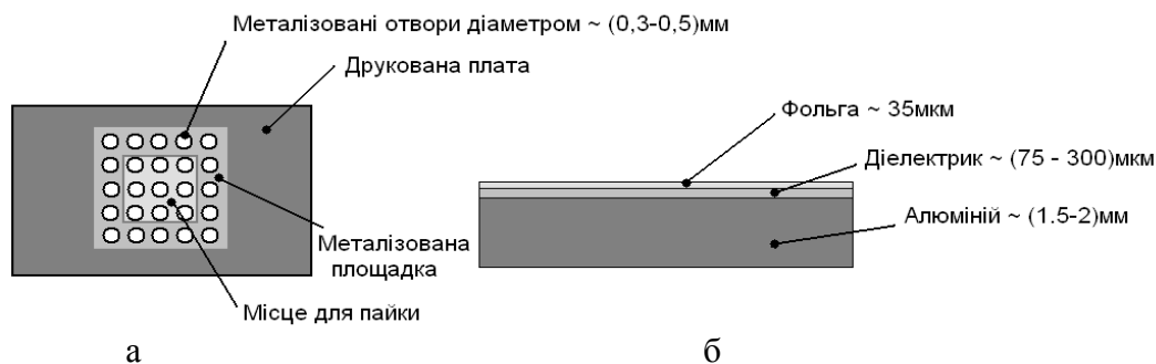
Рис.2. Схематичне зображення друкованої плати з наскрізними отворами (а) та фольгової алюмінієвої плати (б).
